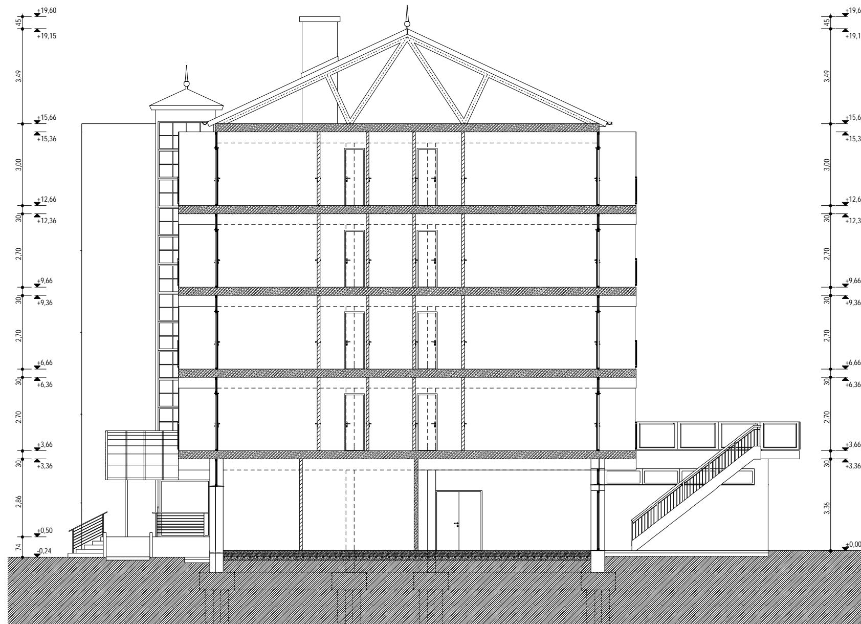
a - a metszet m=1:100
